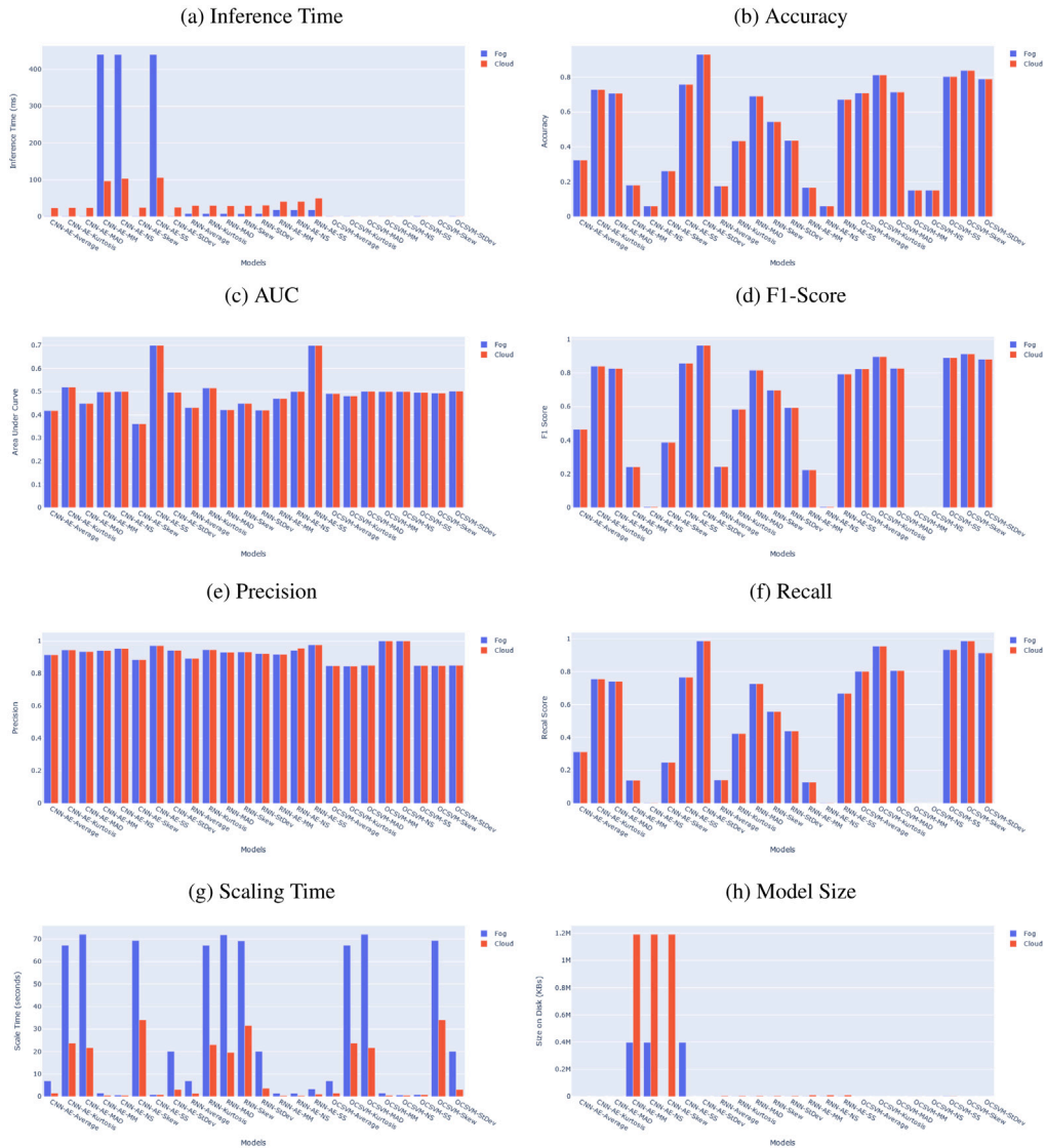
Fig. 10. WADI dataset evaluation.
